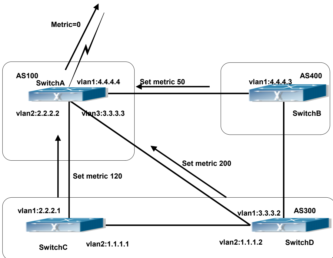
Figure 39-3-4 MED Configuring Topological Map
