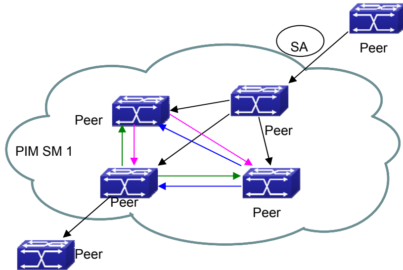
Figure 43-4-2 Flooding of SA messages
